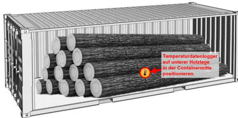
Abb. 2: Messpunkt für die Datenlogger zur Temperaturoaufzeichnung
